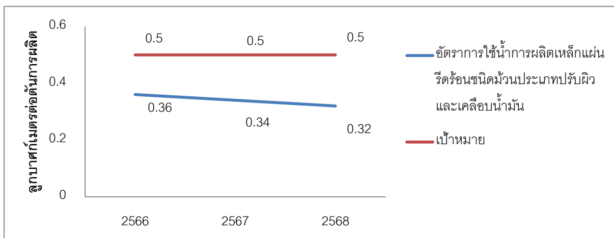
อัตราการใช้น้ำของการผลิตเหล็กแผ่นรีดร้อนชนิดม้วนประเภทลำฉิวและเคลือบน้ำมัน (หน่วย: ลูกบาศก์เมตรต่อตันการผลิต)
